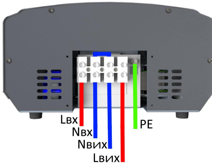
Рисунок 9. Схема підключення до клемної колодки стабілізатора
