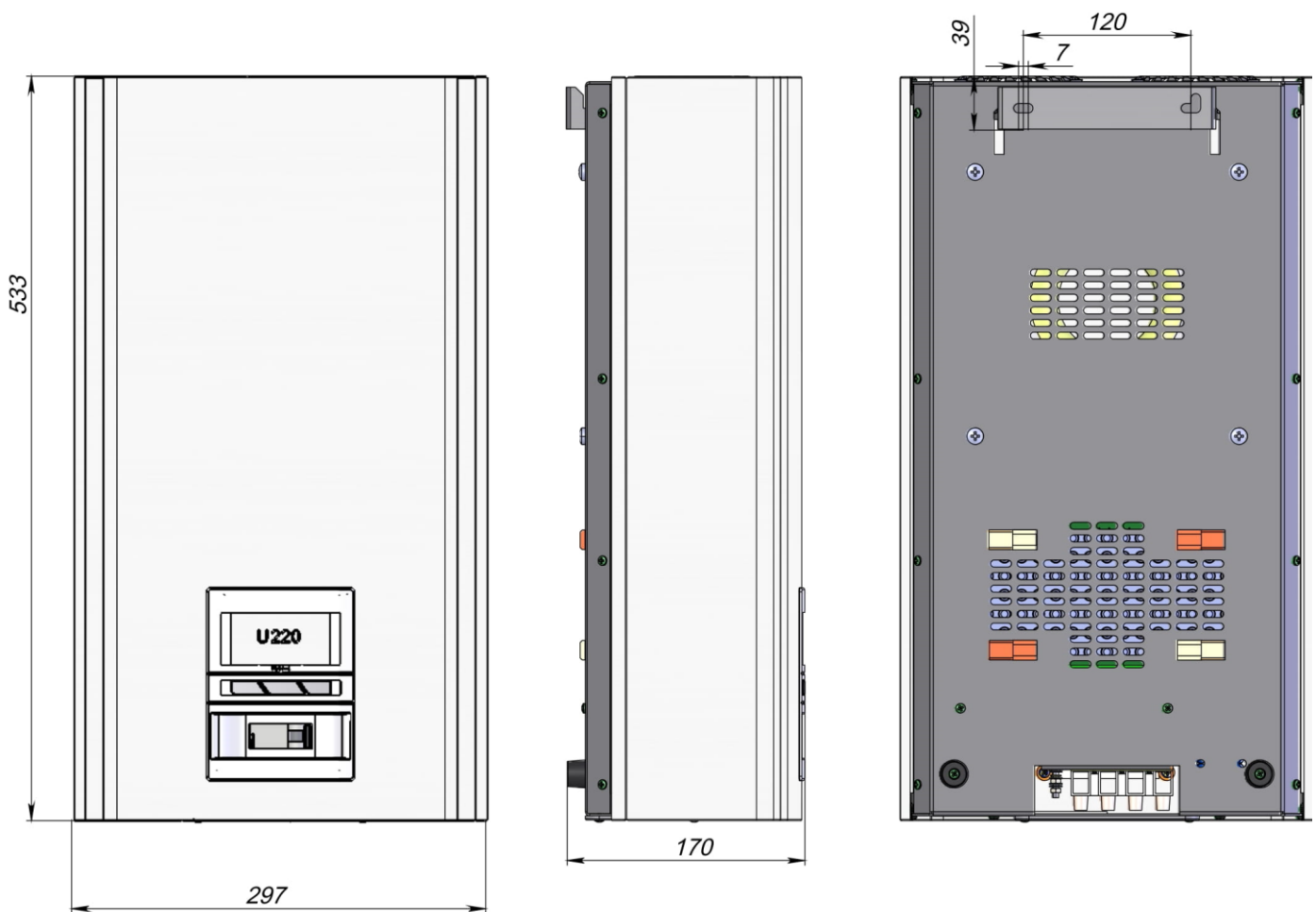
Рисунок 5. Установчі та габаритні розміри стабілізатора
