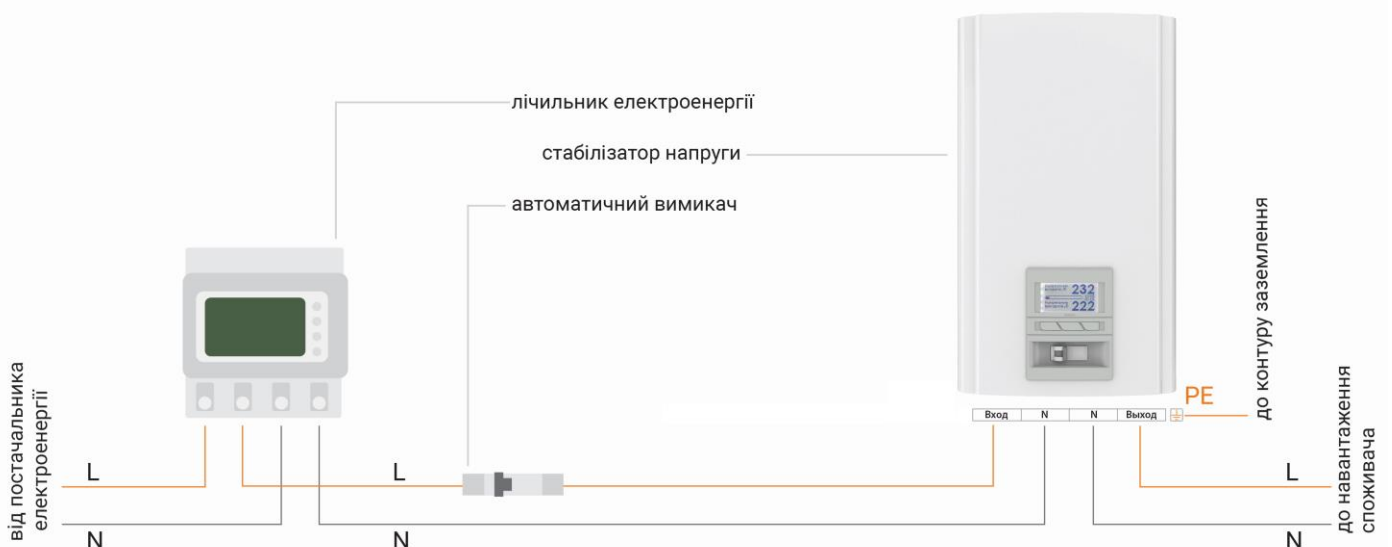
Рисунок 6. Схема підключення стабілізатора КилоГерц до однофазної мережі
