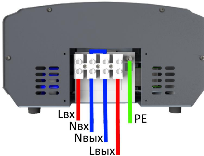
Рисунок 9. Схема подключения к клеммной колодке стабилизатора
