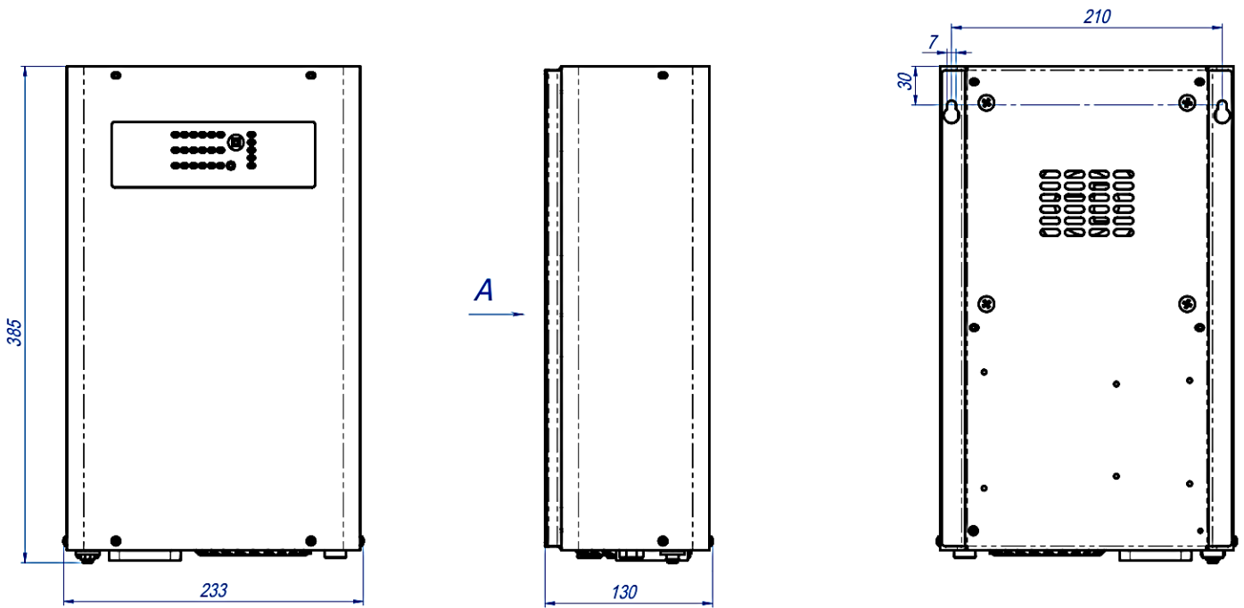
Рисунок 5. Установчі та посадочні розміри ДБЖ
