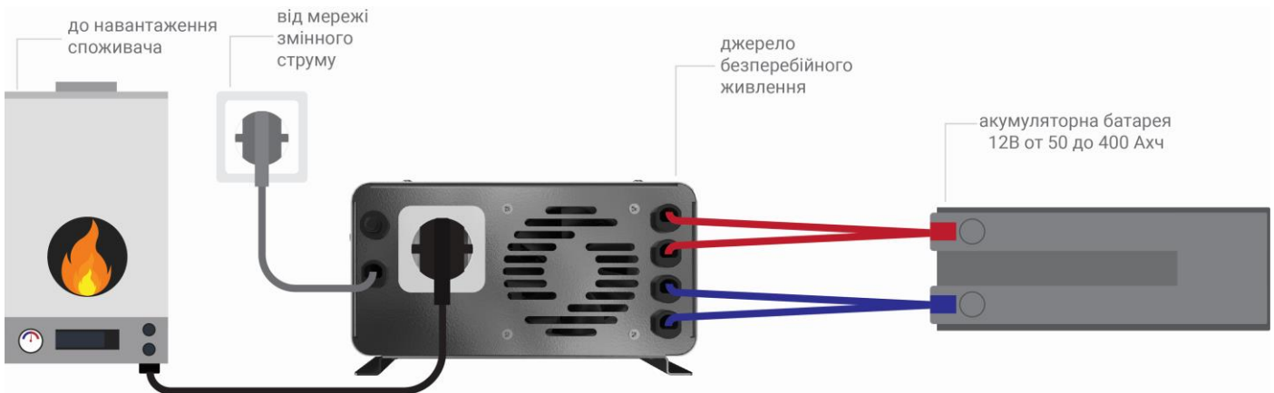
Рисунок 6. Схема підключення ДБЖ до силової мережі
