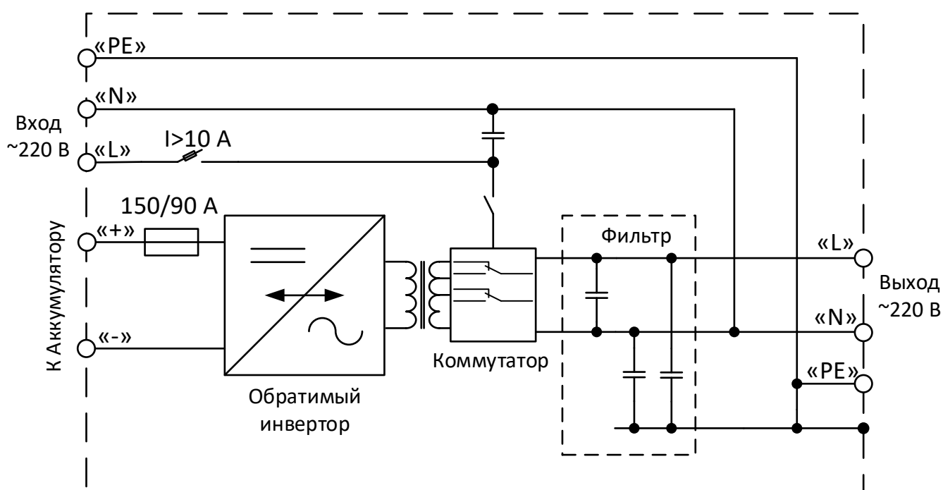
Рисунок 4.Блок-схема ИБП КУЛОН
