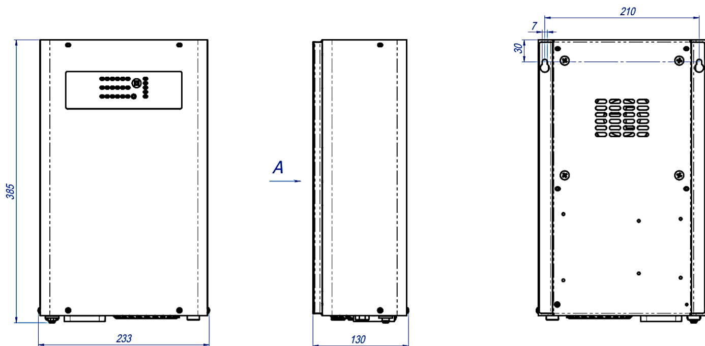
Рисунок 5. Установочные и посадочные размеры ИБП
